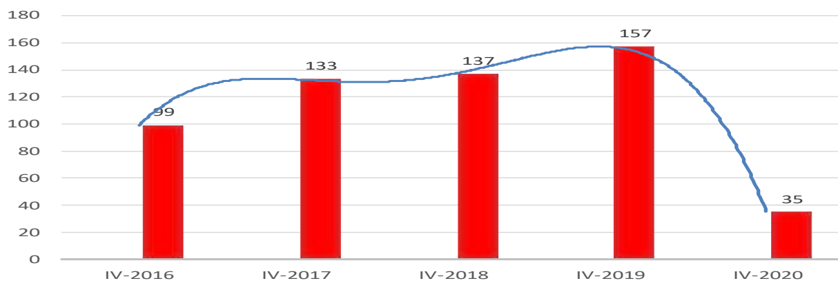
Г.4 Превезени путници у жељезничком саобраћају, 000 G.4 Number of passengers carried in railway transport, 000
